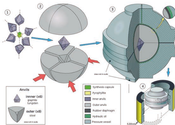
Схема беспрессового аппарата типа разрезная сфера (БАРС)
