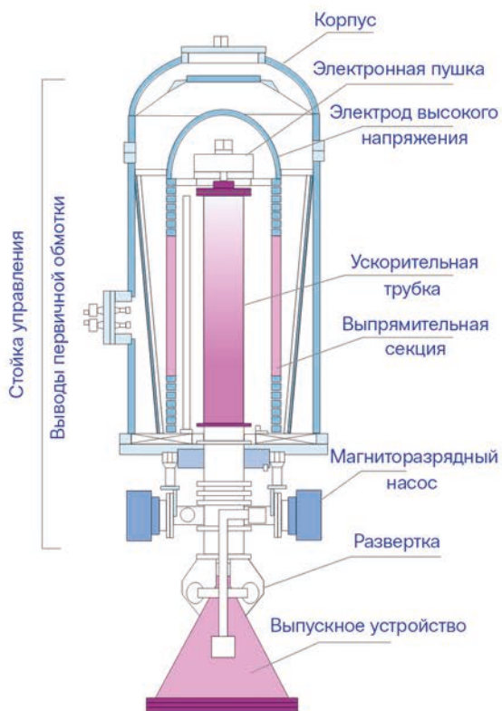
Схема ускорителя электронов ЭЛВ-8
