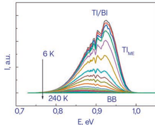
Фотолюминесценции тонкой пленки Cu 2 ZnSnSe 4 в интервале температур 6 – 240 K
