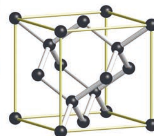
Кристаллическая структура алмаза
