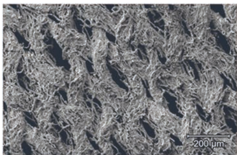
Пористая медная структура, полученная с использованием тканевого темплата
