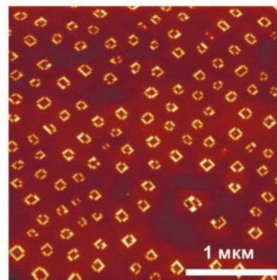
Изображение поверхности упорядоченных квантовых точек Ge в форме прямоугольных колец
