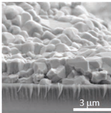
СЭМ изображение поперечного сечения пленки \text{Cu}_2\text{ZnSnSe}_4
