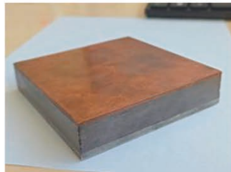
Композиционная сэндвич-структура алюминий — графит — медь
