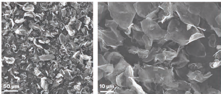
Снимки растровой электронной микроскопии графеновых нанопластинок
