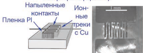
Микроконденсатор
