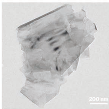
Снимки просвечивающей электронной микроскопии малослойного графена
