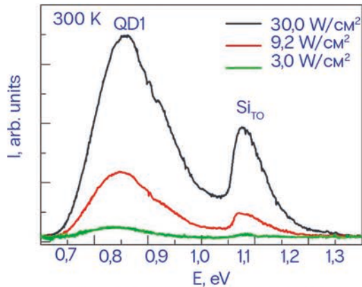
Спектры фотолюминесценции наноструктур Ge/Si с квантовыми точками кольцами Ge, снятые при комнатной температуре ~ 300 K для различной плотности мощности лазерного излучения с \lambda = 532 нм
