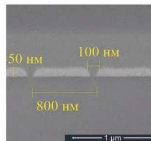
СЭМ изображение поперечного сечения решетки магнито-плазмонных кристаллов после финишного травления
