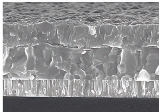
СЭМ-снимок тонкопленочного солнечного элемента
