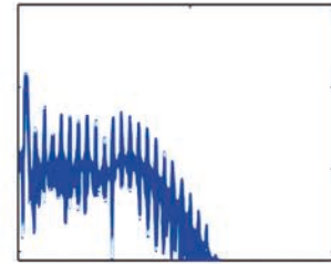
Спектры генерации боковых полос высокого порядка оптомеханической системы
