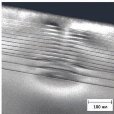
Изображение поперечного сечения многослойной наноструктуры Ge/Si
