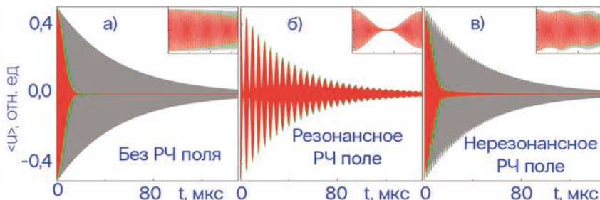
Осцилляции Раби, возбуждаемые однородным (серые линии) и неоднородным (красные и зеленые линии) МВ полем без РЧ поля (а) и с резонансным (б) и нерезонансным (в) РЧ полем
