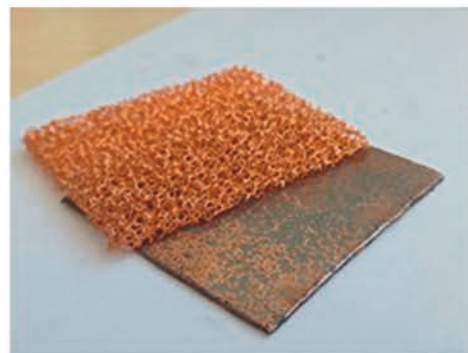
Реструктурированный графит, армированный медной пеной, и исходная медная пена
