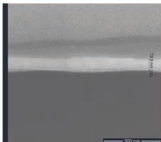
СЭМ изображения поперечного сечения пленки золота на поверхности подложки GaN
