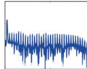
Спектры генерации боковых полос высокого порядка оптомеханической системы
