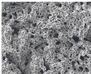
Пористая медная структуру, полученная методом спекания
