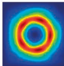
Моделирование прохождения вихревых импульсных пучков в нелинейных средах
