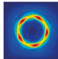
Моделирование прохождения вихревых импульсных пучков в нелинейных средах
