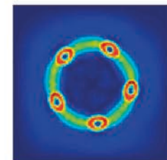
Моделирование прохождения вихревых импульсных пучков в нелинейных средах
