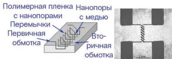
Микротрансформатор
