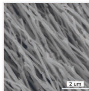
Медные нановолокна
