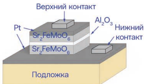
Магниточувствительные многослойные структуры на основе металлоксидных соединений
